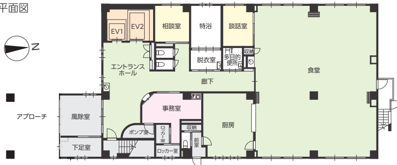
2～4階 平面図
